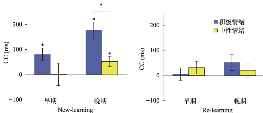
图 4 转换阶段各条件下的背景线索效应
