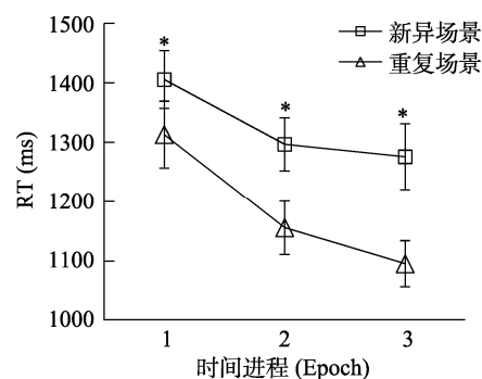
图 3 初始学习阶段每个 epoch 新异场景和重复场景的平均反应时(*表示 p < 0.05 )
