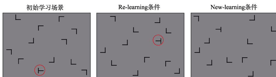
图 1 初始学习阶段和转换阶段的两种学习条件的场景布局
