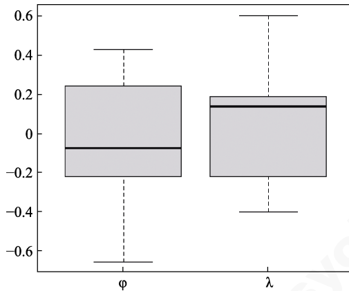
图 5 实证数据中 C-MCDM- \theta 模型的 \varphi_i 和 \lambda_i 估计值分布
