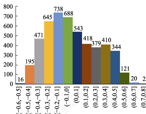
图 2 速度参数分布直方图
