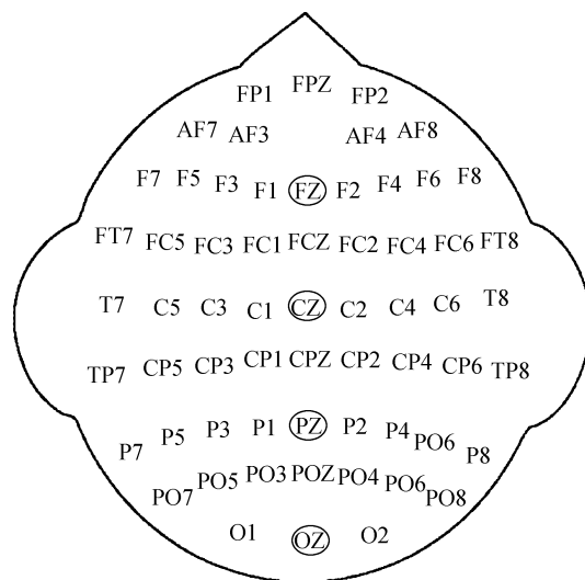
图 2 64 导电极分布
