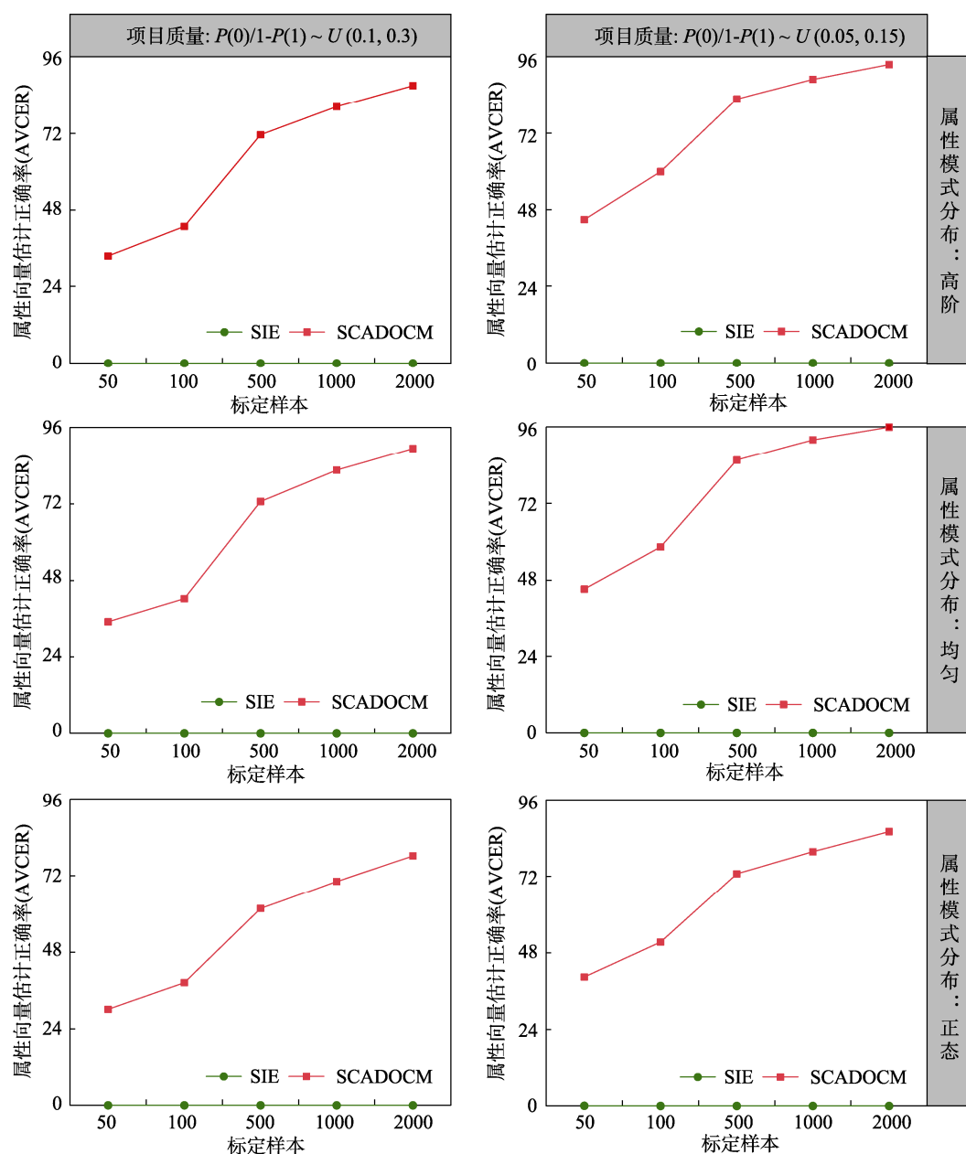
图 2 各在线标定方法在不同条件下的属性向量估计正确率(AVCER)结果
