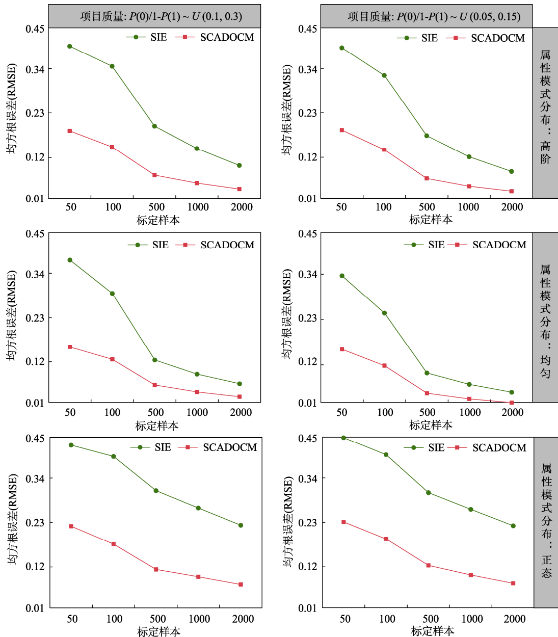
图3 各在线标定方法在不同条件下项目参数标定精度(RMSE)结果
