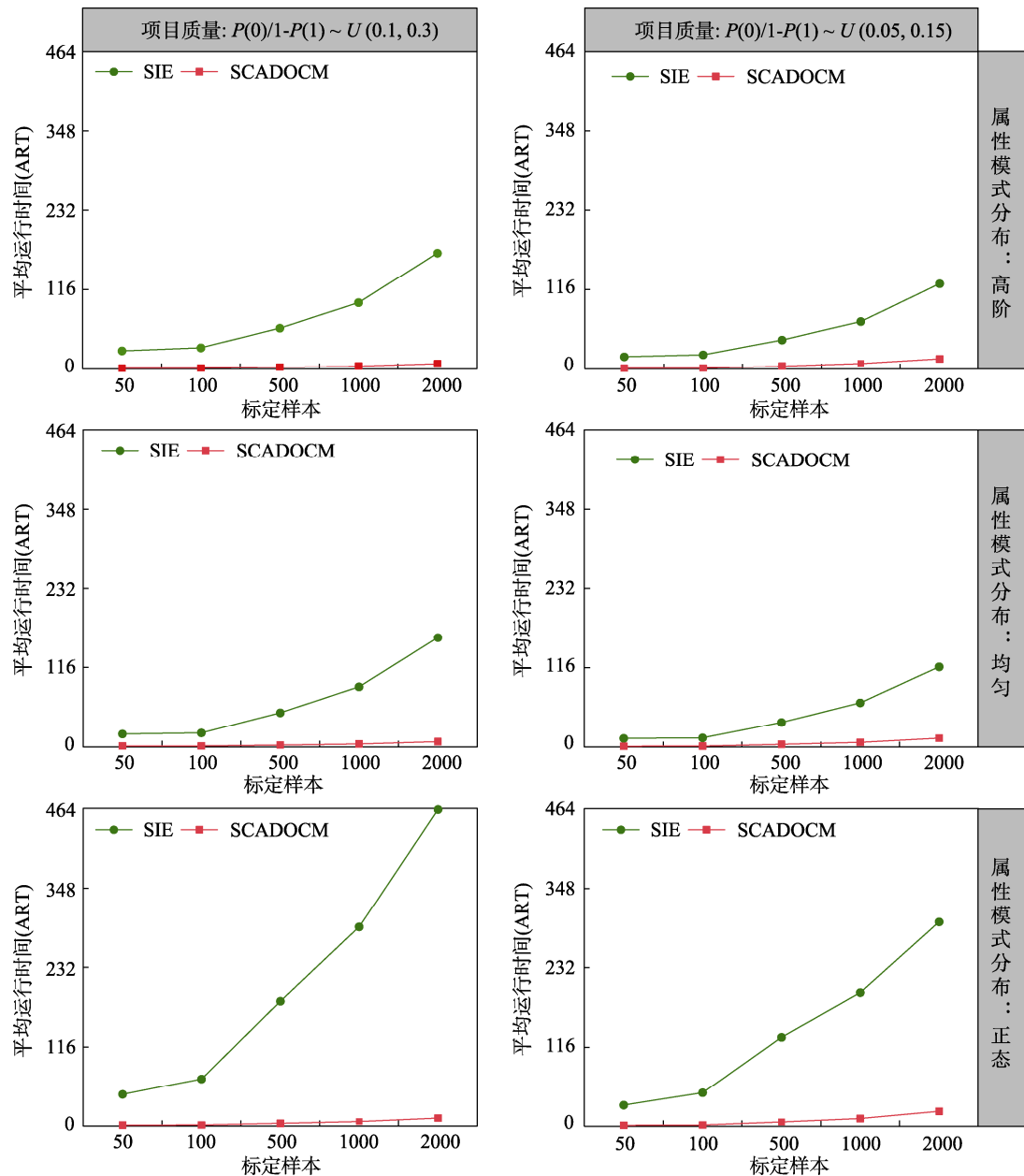
图 1 各在线标定方法在不同条件下的平均运行时间(ART)结果(单位: 秒)
