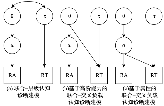
图2 联合-层级和联合-交叉负载认知诊断建模示意图 注: RA = 作答精度; RT = 作答时间; \theta = 能力; \tau = 加工速度; \alpha = 属性。
