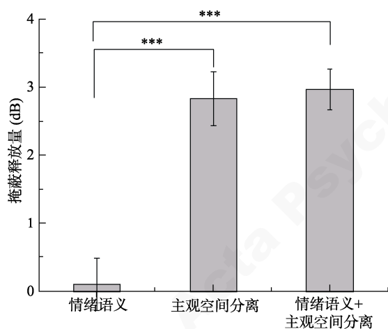
图10 不同线索的掩蔽释放量
