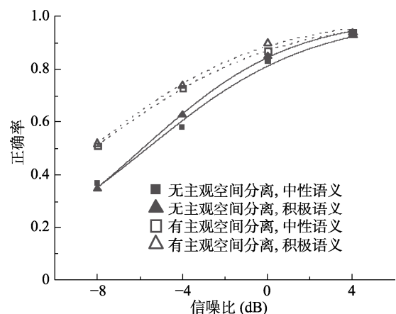
图 8 逆序言语掩蔽下的目标关键词识别正确率
