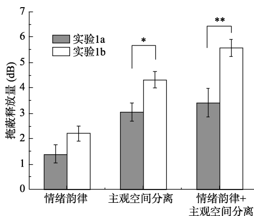
图7 实验1a和实验1b去掩蔽量结果对比
