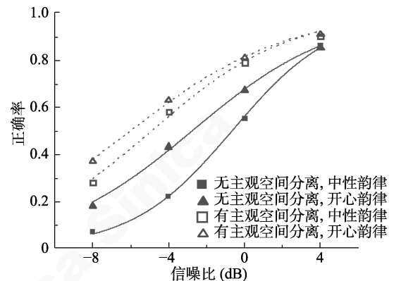
图 4 正序言语掩蔽下目标关键词识别正确率
