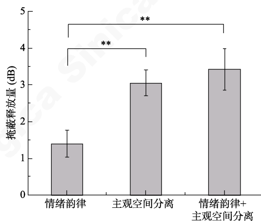
图3 不同听觉线索的掩蔽释放量
