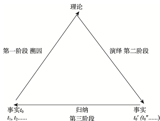
图1 溯因、演绎和归纳的动态循环
