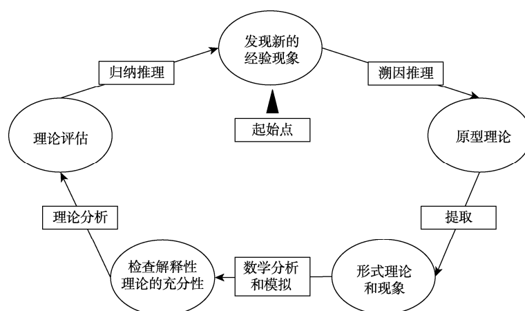
图2 理论建构法理论建构循环图
