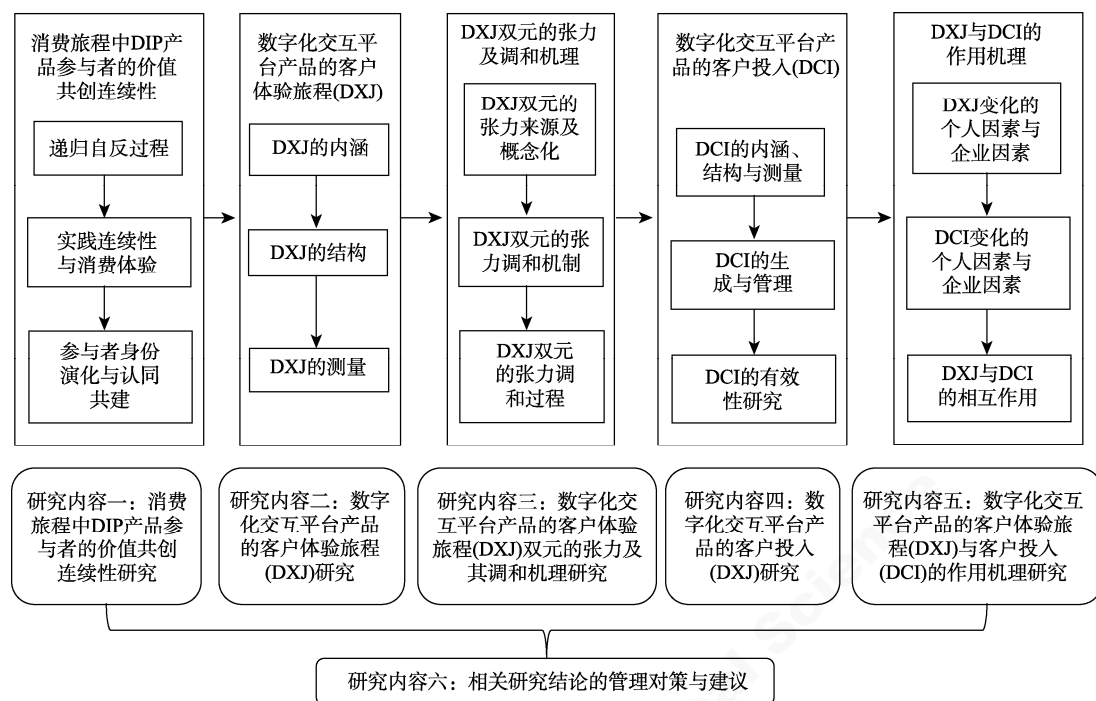
图1 研究框架图
