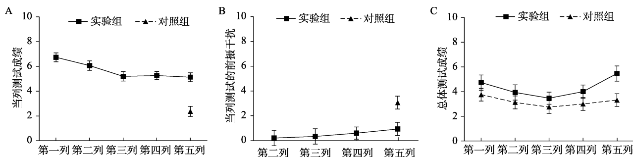
图 3 A: 临时测试在 5 列中的回忆成绩 B: 5 列临时测试中的前摄干扰 C: 最终测试中回忆起的每列的物品量(实验 2) 注: 误差条代表 \pm 1 个标准误
