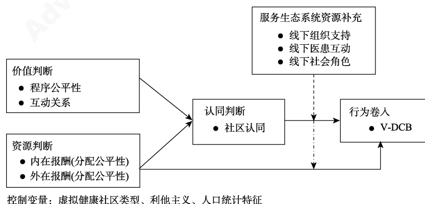
图 1 研究 2 概念模型
