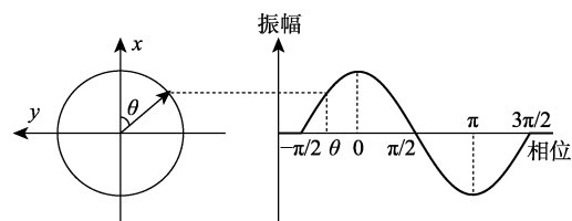
图1 余弦曲线的一个周期及余弦振荡的相位与圆周运动的关系
