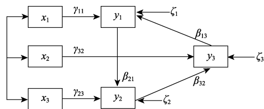
图7 非递归模型
