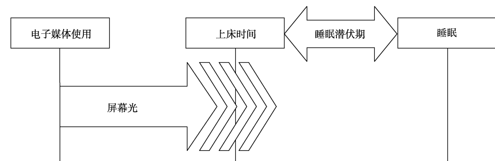
图 4 屏幕光理论
