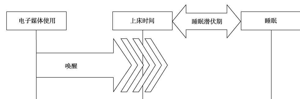
图 3 唤醒理论
